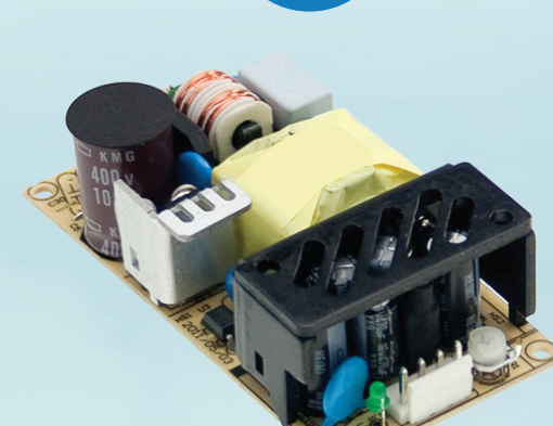
EPS/EPP/PSC系列
