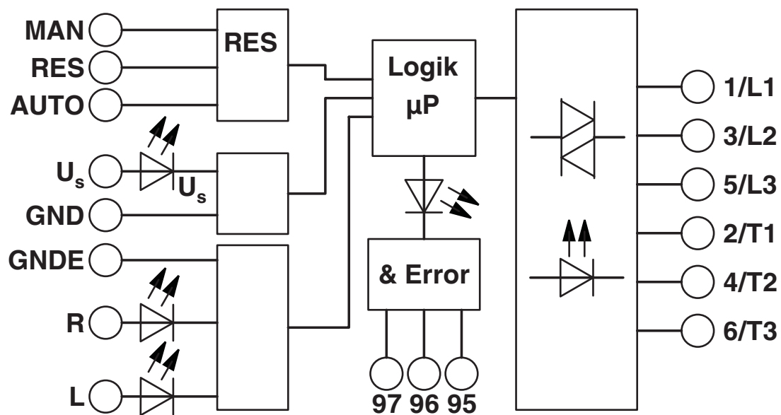
结构框图
